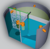
Kleinkläranlagen
